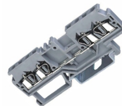
svorkovnice WSxx-QU šedá
