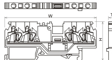
WSxx-DB oranžová
