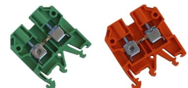
svork. MK4 zelená
