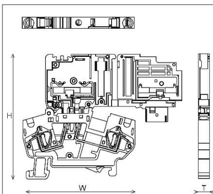
pojistikové pouzdro WSF4-TA
