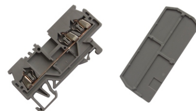
svork. WSxx-TW šedá bočnice D-WSxx-TW
